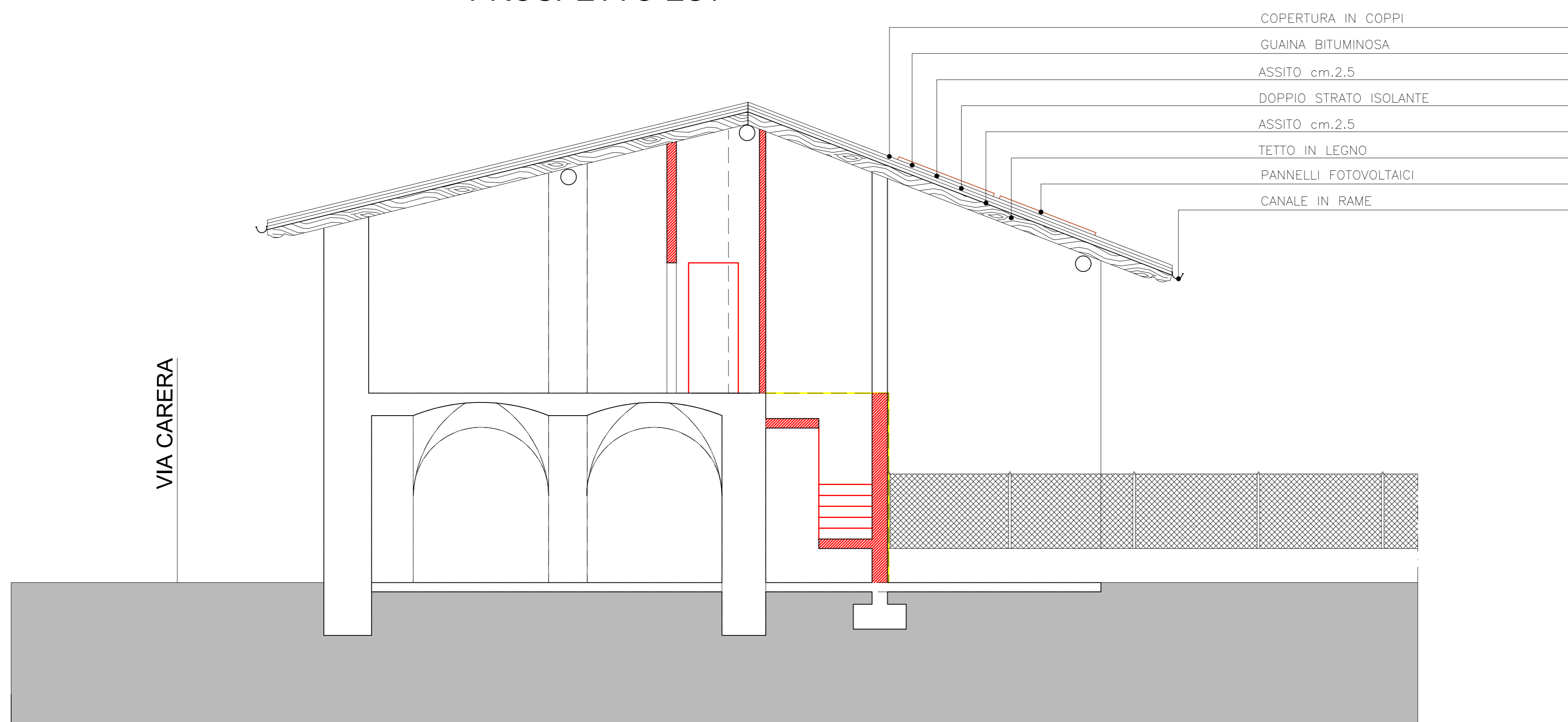
PROSPETTO EST
