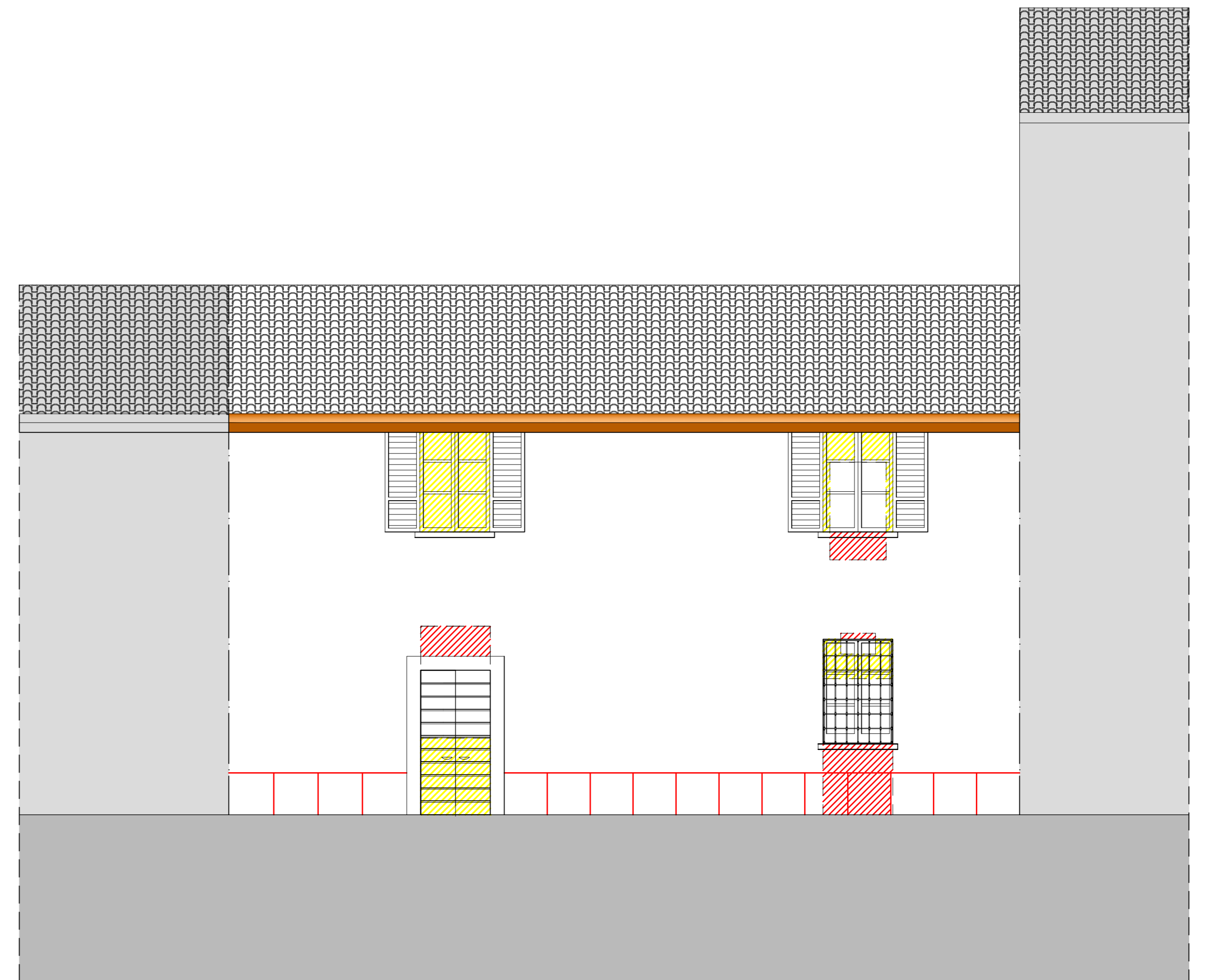
PROSPETTO OVEST
