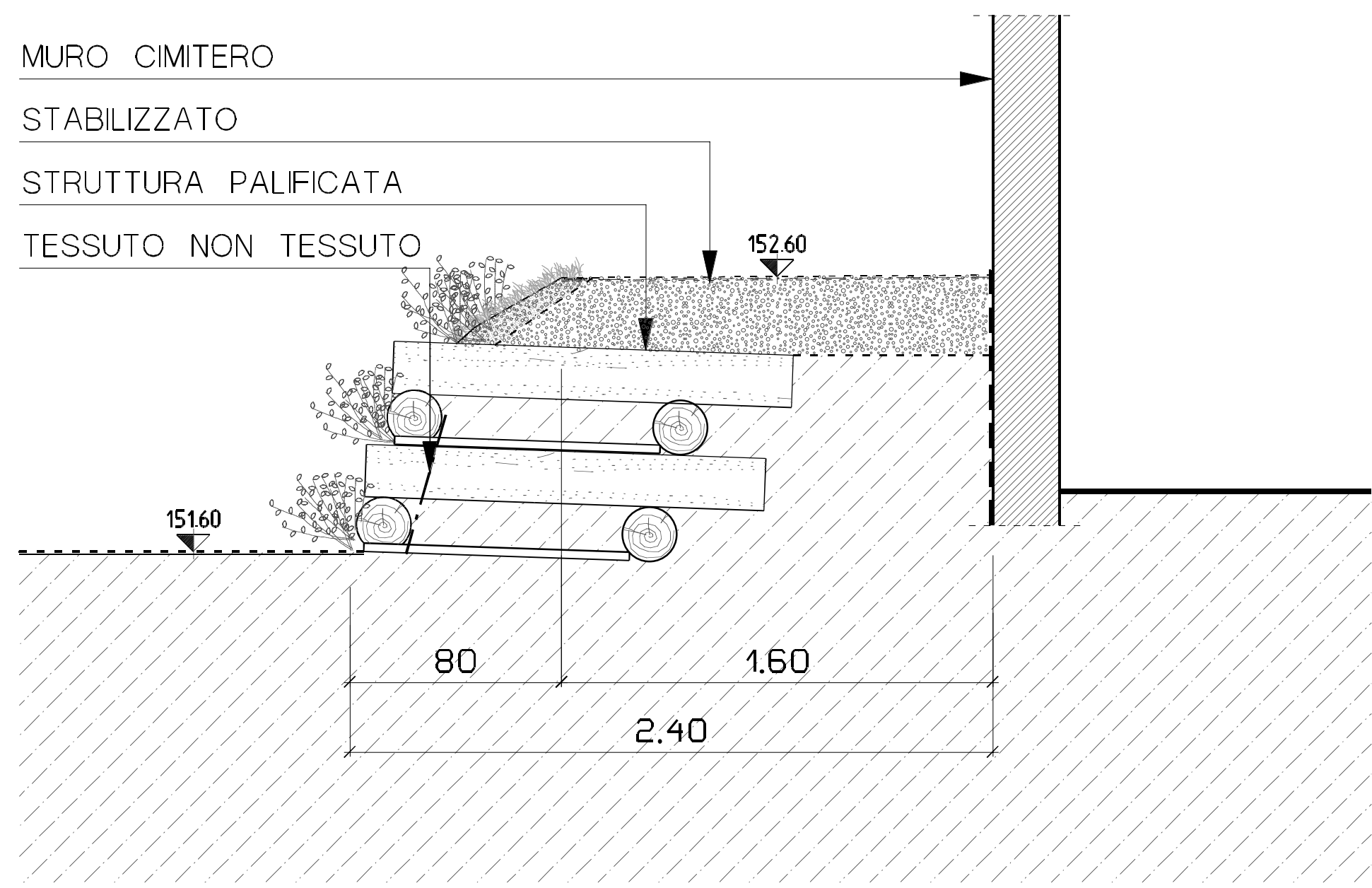
SEZIONE A-A IN PROGETTO - Scala 1:20
