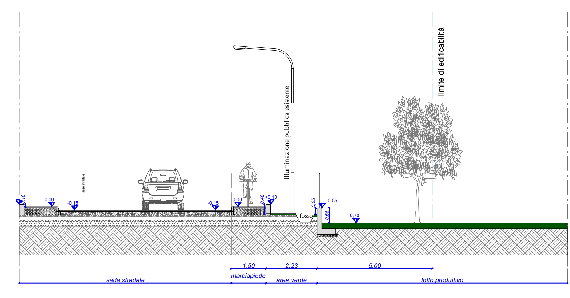
SEZIONE A:A Scala disegno 1: 100
