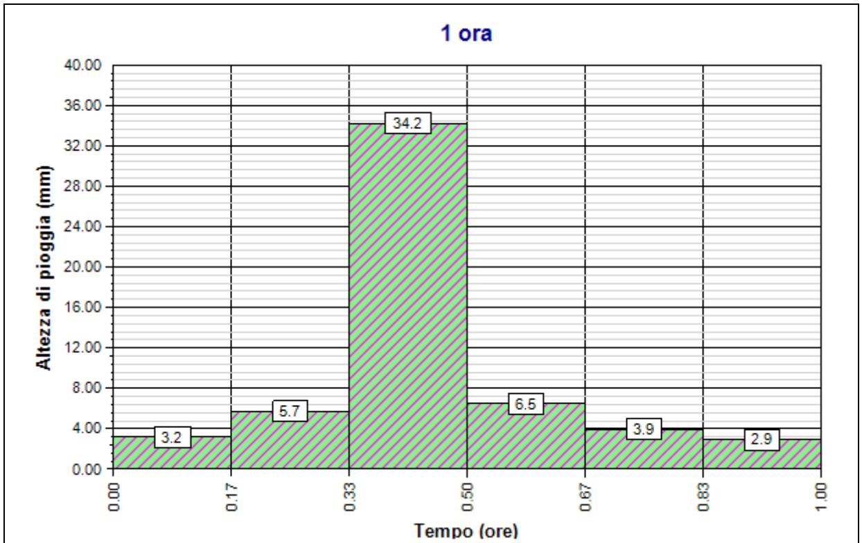
Figura 5 - Ietogramma Chicago piogge inferiori a 1 ora
