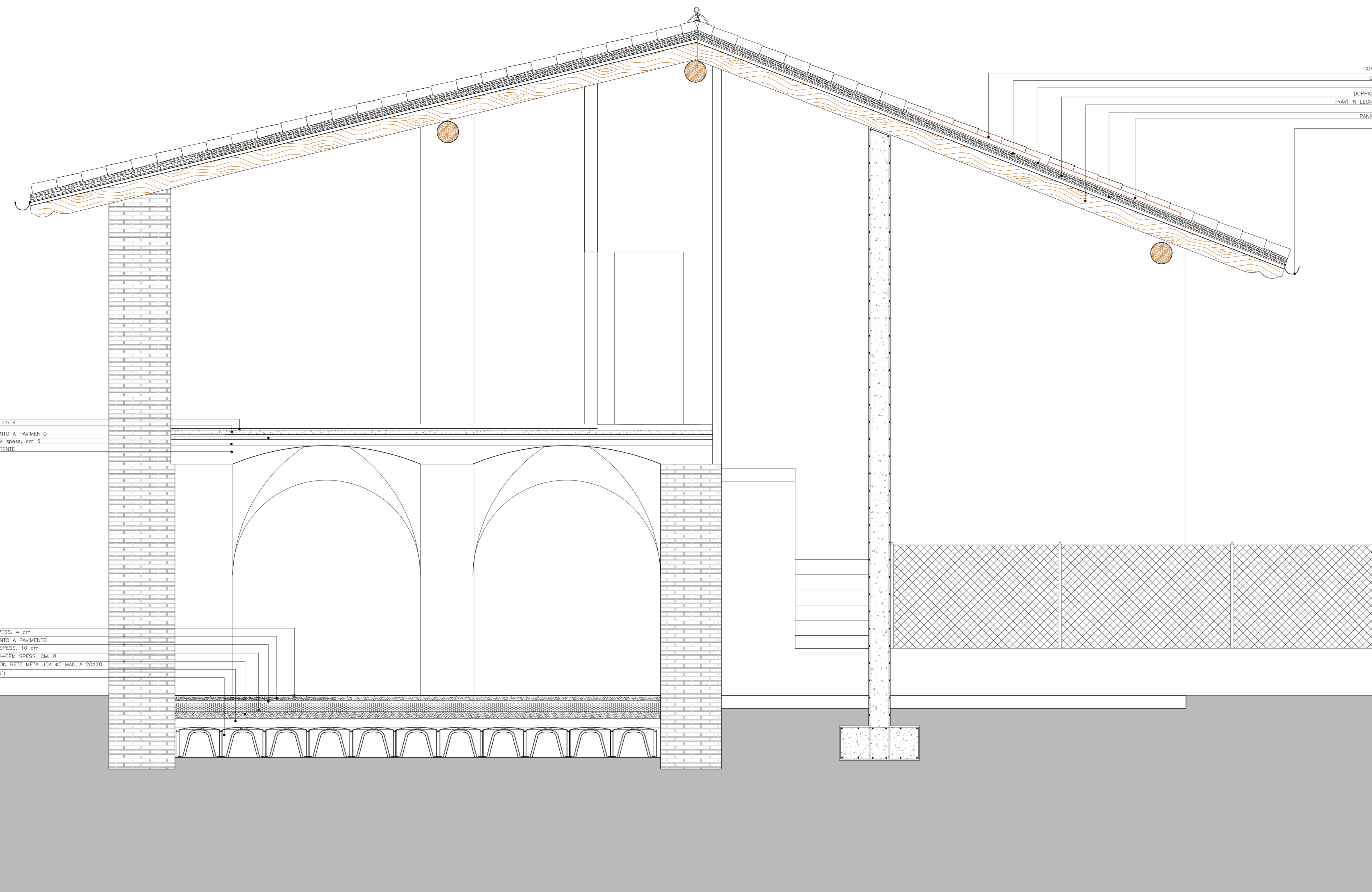
SEZIONE A-A
